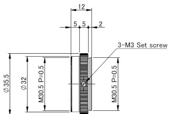
代替提案品：FASV-PLA305-RS
